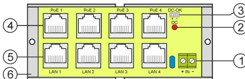
Rys. 2. Rozmieszczenie elementów.
