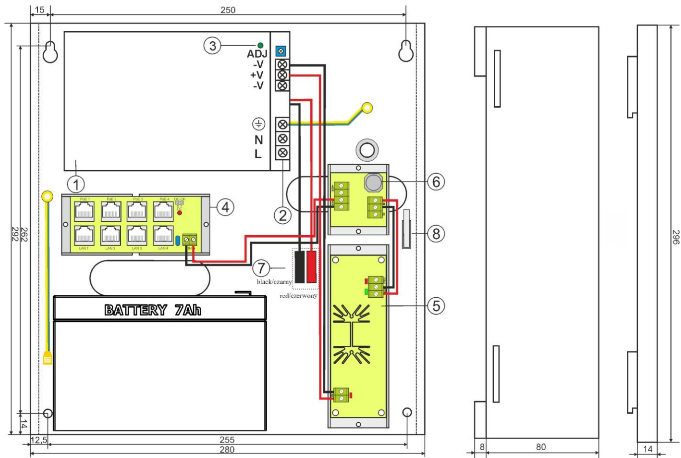
Rys. 3. Widok zasilacza.
